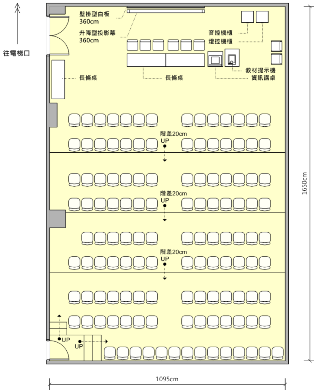
圖 3 視聽教室 A 平面圖(高中組、國中組)
